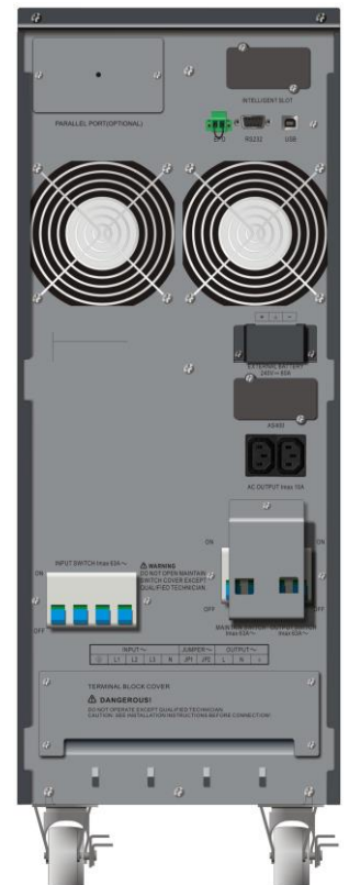
VFI 20000 TP
